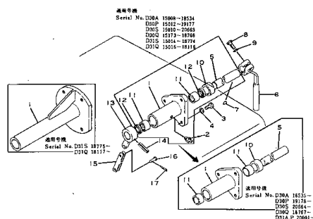
コンプレッション リリース レバー Fig. 2103 COMPRESSION RELEASE LEVER
