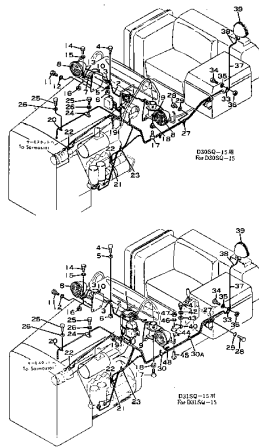
ヘッド ランプ および ワイヤリング Fig. 2143 HEAD LAMP AND WIRING (D30.31 S,Q-15)
