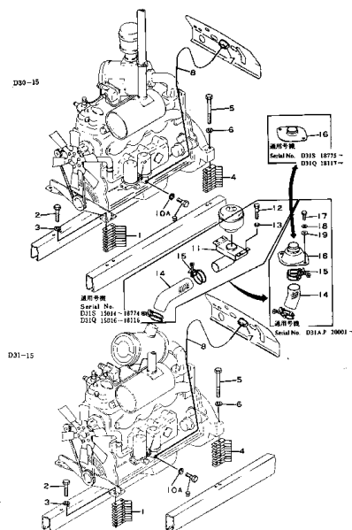
エンジン関連部品 Fig. 2101 ENGINE RELATED PARTS
