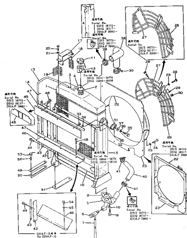
ラジエーター Fig. 2122 RADIATOR (D31-15)
