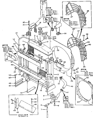
Fig. 2122 RADIATOR (D31-15)
