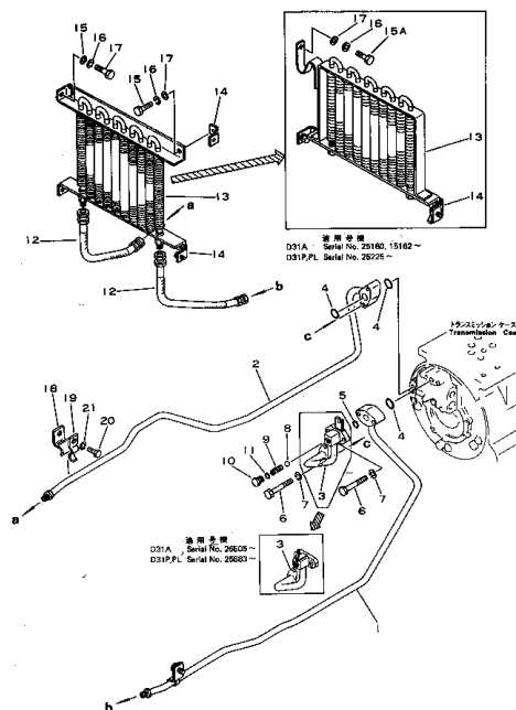
オイルクーラおよびパイピング (適用機種) Fig. 3135A OIL COOLER AND PIPING (Serial No. 25003~)
