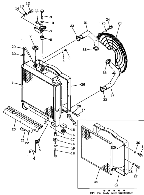
ラジエータ および パイピング Fig. 3131 RADIATOR AND PIPING
