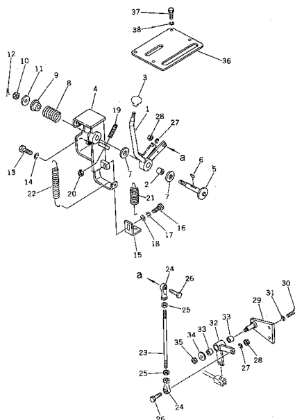
フュエルコントロールレバー Fig. 121 FUEL CONTROL LEVER
