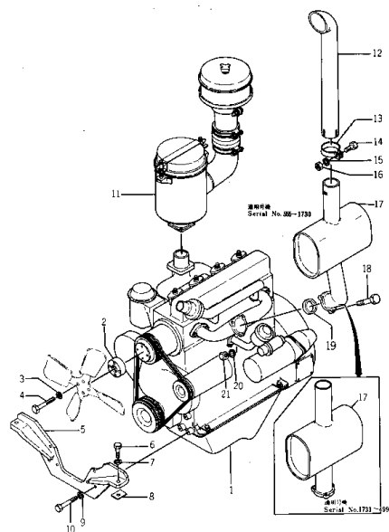
エンジン関連部品 (適用号機) Fig. 101 ENGINE RELATED PARTS (Serial No. 555~4999)
