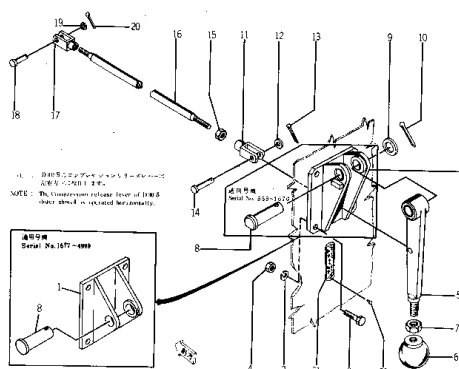
Fig. 105 コンプレッション リリース レバー (適用号 555~4999) Fig. 105 COMPRESSION RELEASE LEVER (Serial No. 555~4999)
