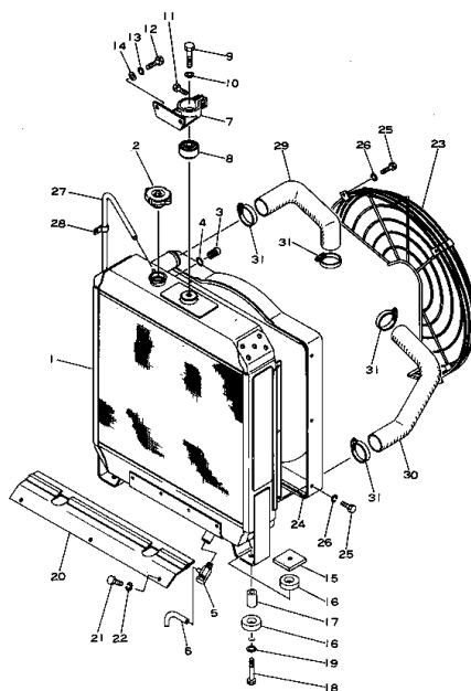
ラジエーター および パイピング Fig. 3131 RADIATOR AND PIPING
