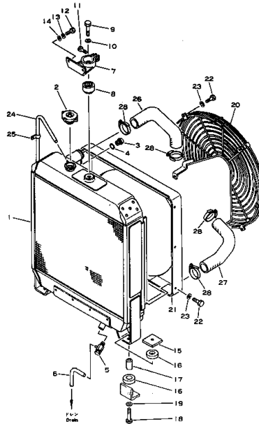
ラジエータ および パイピング Fig. 3131 RADIATOR AND PIPING
