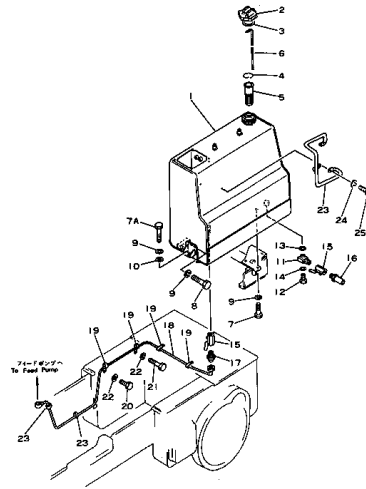
Fig. 3141 フュエル タンク および パイピング FUEL TANK AND PIPING (適用機種) (D30SF Serial No. 26967~28000) (D30QF Serial No. 26955~28000)
