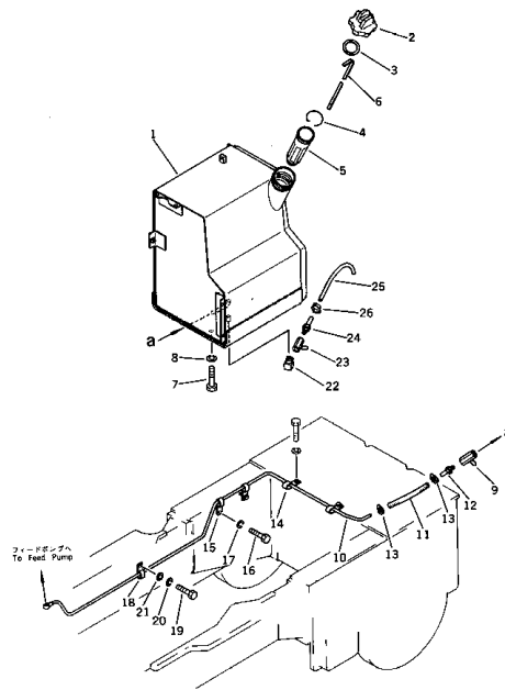
フエール タンク およびパイピング Fig. 141 FUEL TANK AND PIPING
