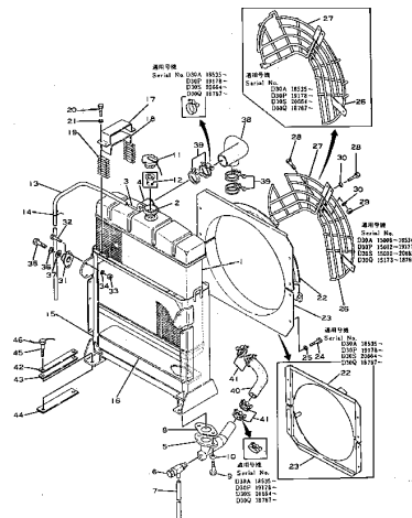
ラジエーター Fig. 2121 RADIATOR (D30-15)
