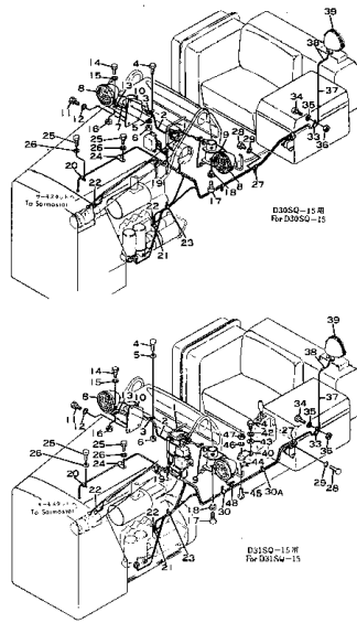
ヘッド ランプ および ワイヤリング Fig. 2143 HEAD LAMP AND WIRING (D30,315,Q-15)
