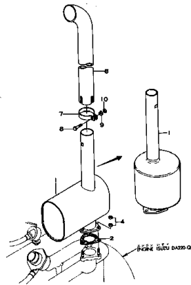
エキゾースト マフラー Fig. 1123 EXHAUST MUFFLER
