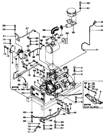
Fig. 1101 エンジン関連部品 (D30S.Q Serial No. 5004~)
