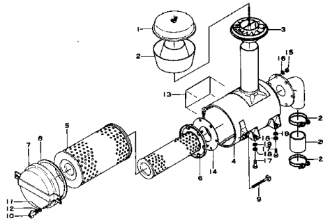
Fig. 1103 エアークリーナ AIR CLEANER
