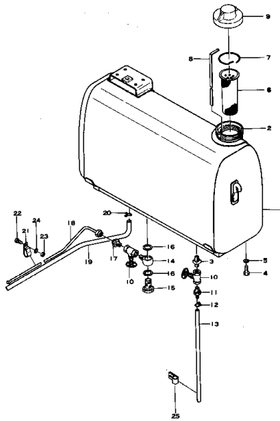
Fig. 1122 FUEL TANK AND PIPING フュエル タンク および パイピング
