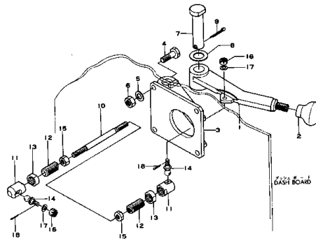
コンプレッション リリース レバー Fig. 1105 COMPRESSION RELEASE LEVER
