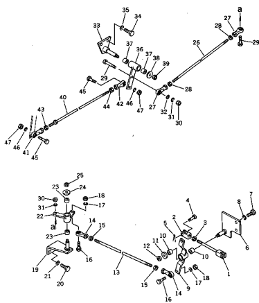
フェュエルコントロール リンケージ Fig. 122 FUEL CONTROL LINKAGE
