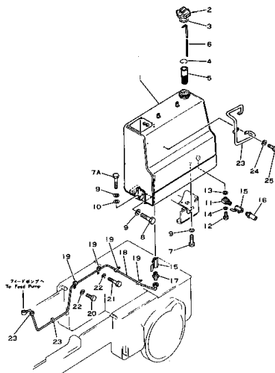
Fig. 3141 フュエル タンク および パイピング FUEL TANK AND PIPING 適用機種 (D30AF Serial No. 25633 ~ 28000) (D30PF Serial No. 25766 ~ 28000)
