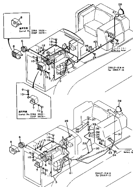
ヘッド ランプ および ワイヤリング Fig. 2142 HEAD LAMP AND WIRING (D30,31 A,P-15)
