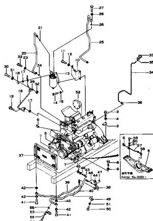
エンジン関連部品 Fig. 1102 ENGINE RELATED PARTS (D30A, P Serial No. 5004-)
