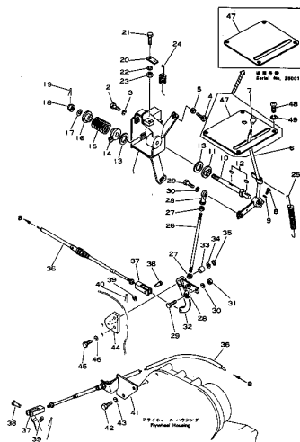
Fig. 3121 燃料コントロールレバー FUEL CONTROL LEVER
