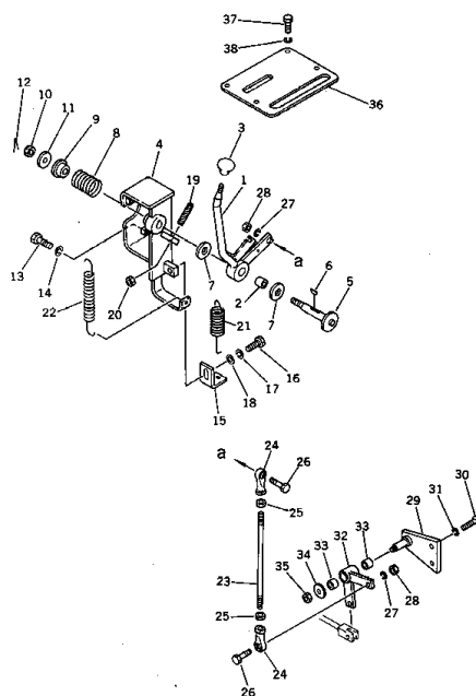
Fig. 121 FUEL CONTROL LEVER フュエルコントロールレバー
