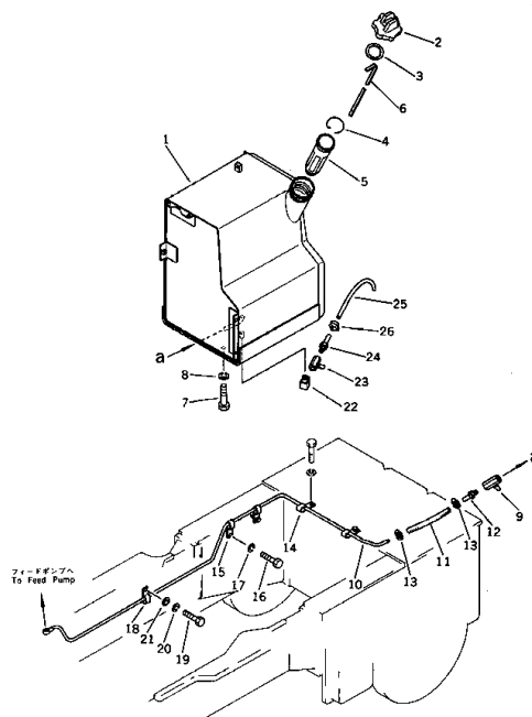
フュエル タンク およびパイピング Fig. 141 FUEL TANK AND PIPING
