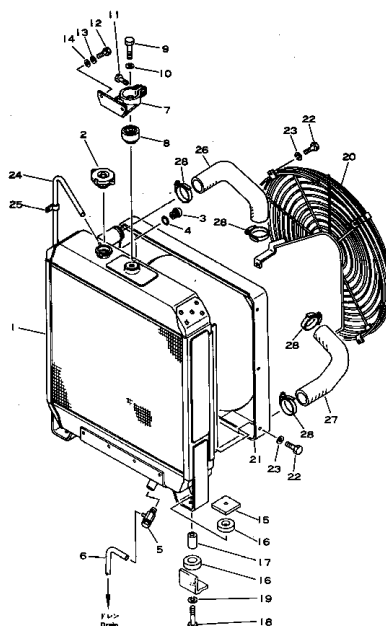
ラジエーター および パイピング Fig. 3131 RADIATOR AND PIPING
