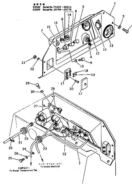
Fig. 3155 インストルメント パネル INSTRUMENT PANEL
