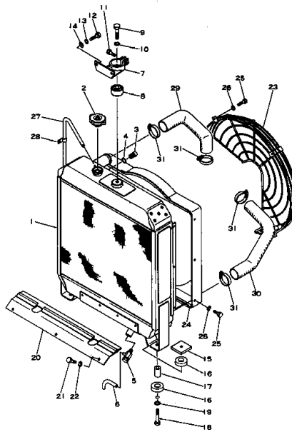
ラジエータ および パイピング Fig. 3131 RADIATOR AND PIPING
