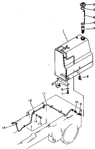
Fig. 3141A フュエル タンク および パイピング FUEL TANK AND PIPING 適用機種 (D30AF Serial No. 28001~) (D30PF Serial No. 28001~)
