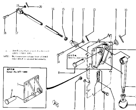
Fig. 105 コンプレッション リリース レバー (適用 号 機 (Serial No. 555~4999))
