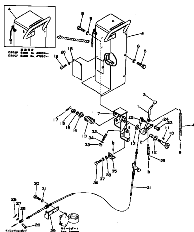
Fig. 2121 FUEL CONTROL LEVER フエエル コントロール レバー
