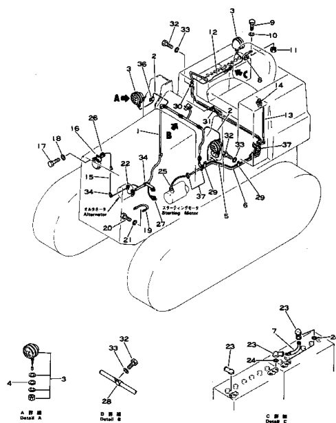
エレクトリカル システム Fig. 2161 ELECTRICAL SYSTEM
