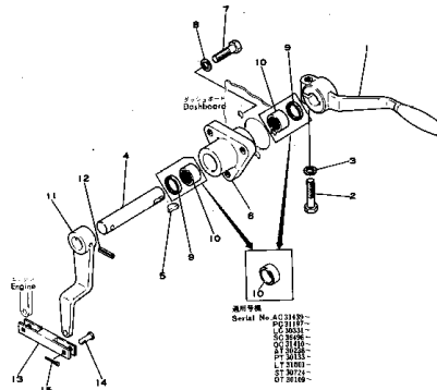
コンプレッション リリーズ レバー Fig. 1103 COMPRESSION RELEASE LEVER
