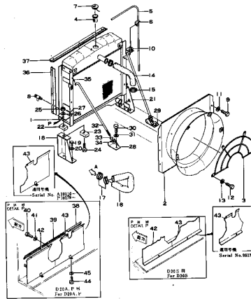
Fig. 123A RADIATOR (Serial No. D20A,SP 4365--)
