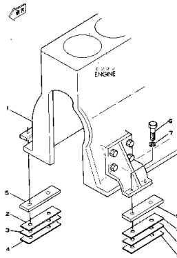
エンジン アタッチング パーツ Fig. 101 ENGINE ATTACHING PARTS
