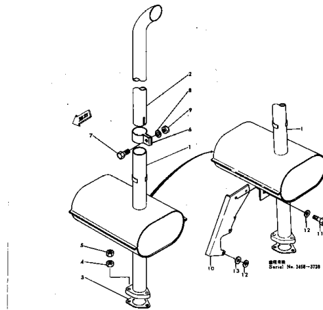
エキゾースト マフラー (適用機種 Serial No. 1005~3728) Fig. 122 EXHAUST MUFFLER (Serial No. 1005~3728)
