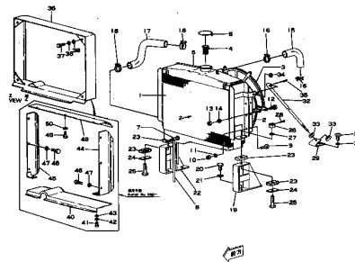
ラジエーター (散热器) Fig. 123 RADIATOR (Serial No. D20A,S 7~4364)
