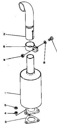
エキゾースト マフラー (部品番号) Fig. 122A EXHAUST MUFFLER (Serial No. 3729~)
