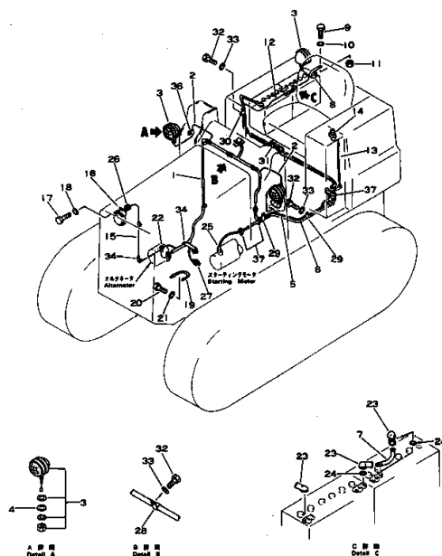
Fig. 2161 エレクトリカル システム ELECTRICAL SYSTEM
