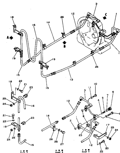
オイル クーラ および パイピング Fig. 2135 OIL COOLER AND PIPING
