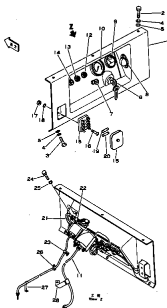
インスツルメント パネル Fig. 2155 INSTRUMENT PANEL
