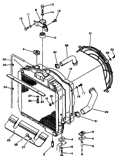
ラジエータ および パイピング Fig. 2131 RADIATOR AND PIPING
