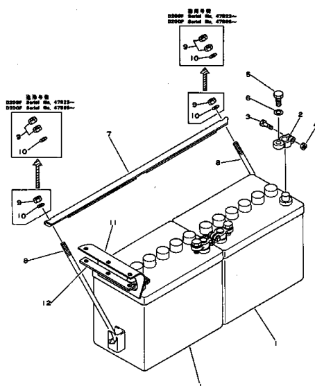
Fig. 2151 バッテリー BATTERY
