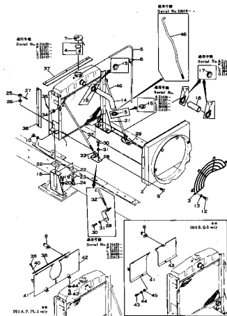
ラジエーター Fig. 1121 RADIATOR (D20-3)
