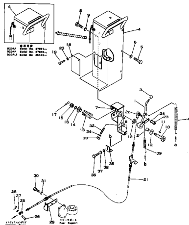
Fig. 3121 フューエル コントロール レバー FUEL CONTROL LEVER
