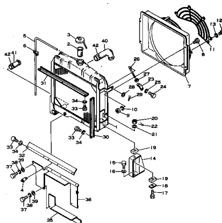
ラジエータ Fig. 1121 RADIATOR
