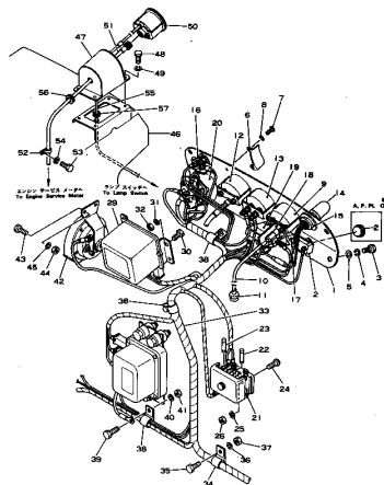
インストルメント パネル レギュレータ および ヒューズ ボックス Fig. 1141 INSTRUMENT PANEL REGULATOR AND FUSE BOX
