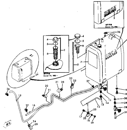
Fig. 127 FUEL TANK AND PIPING (適用 機種 Serial No. 1005~)
