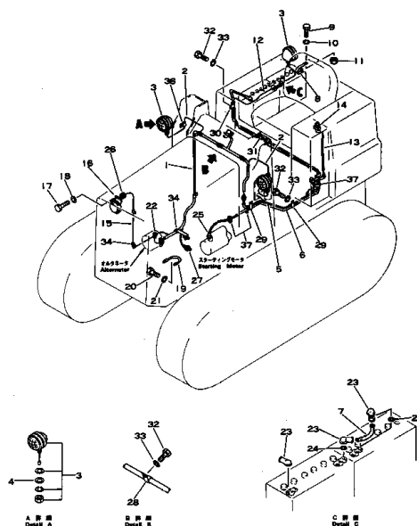
Fig. 3161 エレクトリカル システム ELECTRICAL SYSTEM
