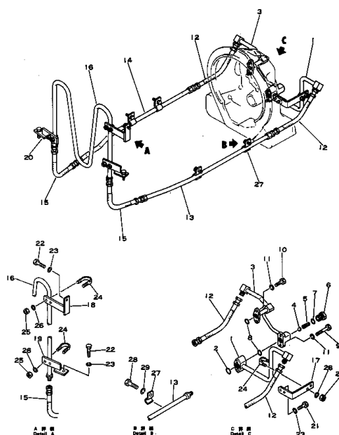
オイル クーラ および パイピング Fig. 3135 OIL COOLER AND PIPING
