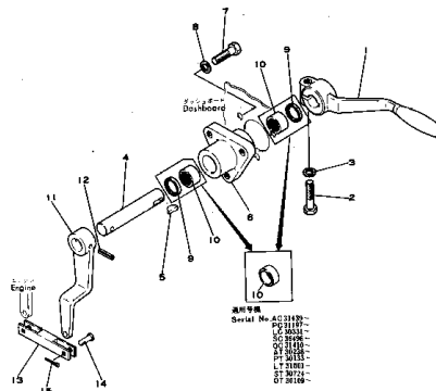
コンプレッション リリース レバー Fig. 1103 COMPRESSION RELEASE LEVER
