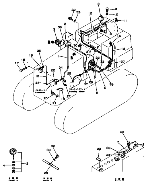
Fig. 3161 エレクトリカル システム ELECTRICAL SYSTEM
