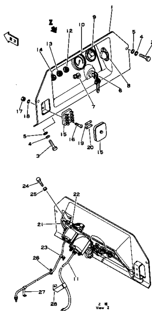
インスツルメント パネル Fig. 3155 INSTRUMENT PANEL
