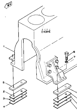
エンジン アタッチング パーツ Fig. 101 ENGINE ATTACHING PARTS
