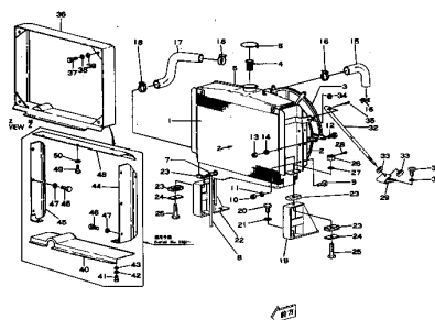
ラジエーター 図 123 Fig. 123 RADIATOR (Serial No. D20A,S 7~4364)
