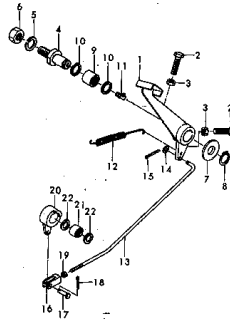
デクセルペダル (トルクフロー式) Fig. 1109 DECELERATOR PEDAL (Torqflow Drive)
