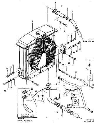
ラジエーター関連部品 (適用車種) Fig. 1121 RADIATOR RELATED PARTS (Serial No. 2501~3344)
