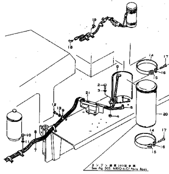
バイパス フィルタ および ブラケット Fig. 1104 BYPASS FILTER AND BRACKET
