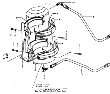
バイパス フィルタ ブラケット Fig. 1103 BYPASS FILTER BRACKET
