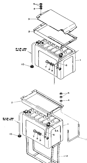
Fig. 141 バッテリー BATTERY
