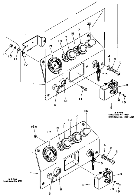
インスツルメント パネル Fig. 145 INSTRUMENT PANEL
