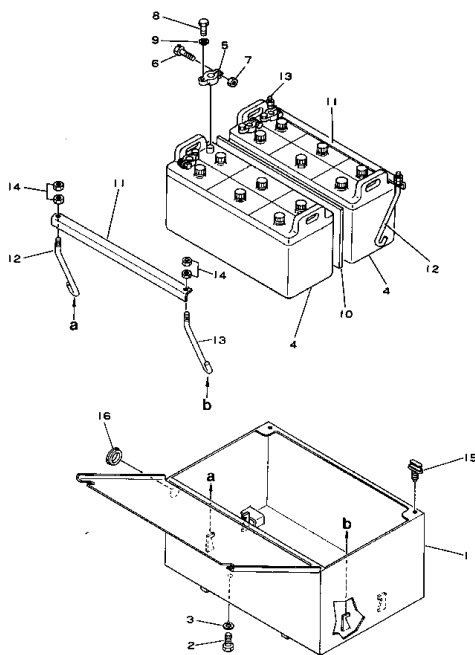
Fig. 151 バッテリー BATTERY
