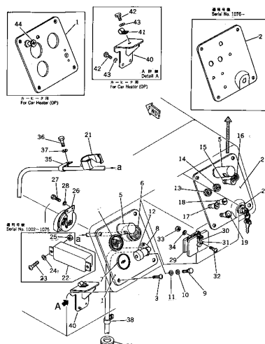
Fig. 155 インストルメント パネル INSTRUMENT PANEL
