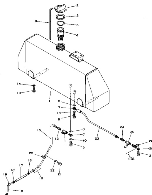
Fig. 141 フュエル タンク FUEL TANK
