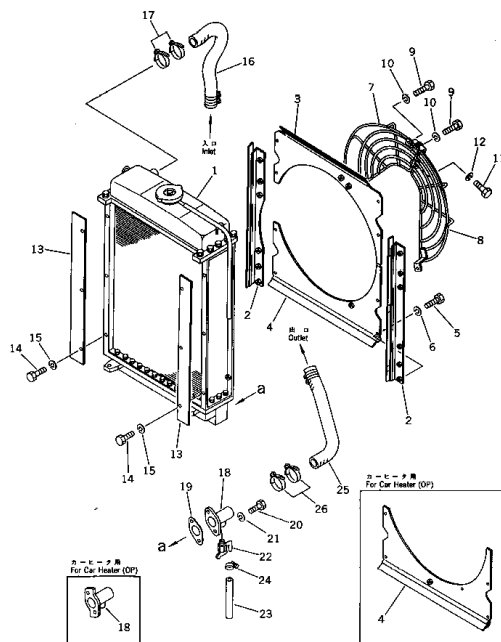
Fig. 132 ラジエータ カバー および パイピング RADIATOR COVER AND PIPING
