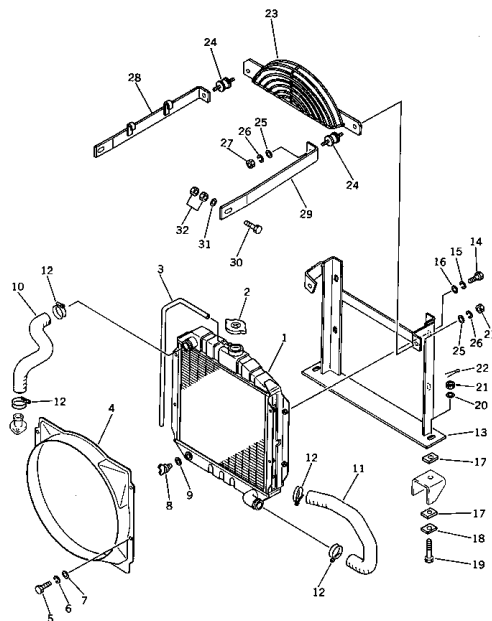
ラジエータ Fig. 131A RADIATOR (適用号数) (Serial No. 1191~)
