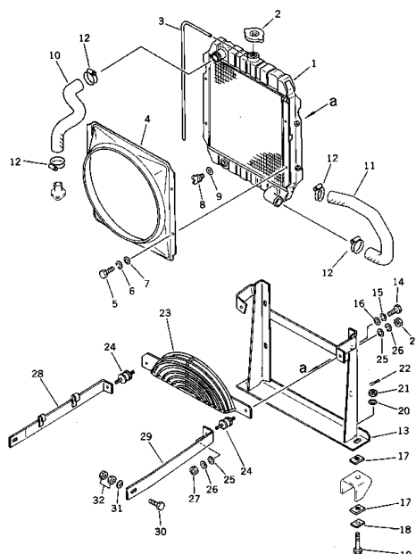
ラジエータ Fig. 131 RADIATOR (適用号機) (Serial No. 1001-1190)
