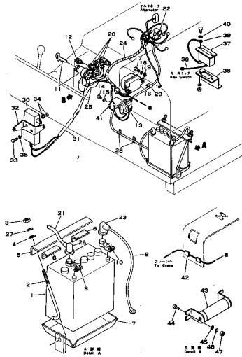
エレクトリカル システム Fig. 162 ELECTRICAL SYSTEM (CD25C)
