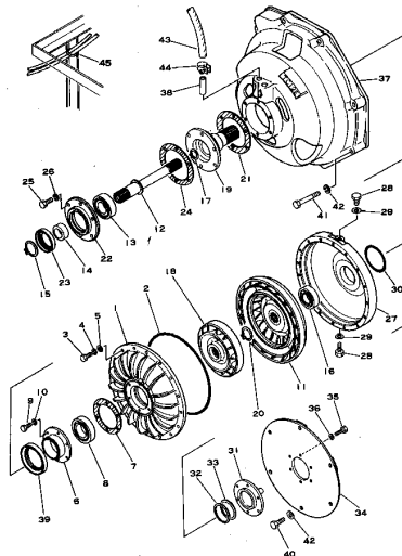
トルクコンバータ Fig. 222 TORQUE CONVERTER (CD25C)
