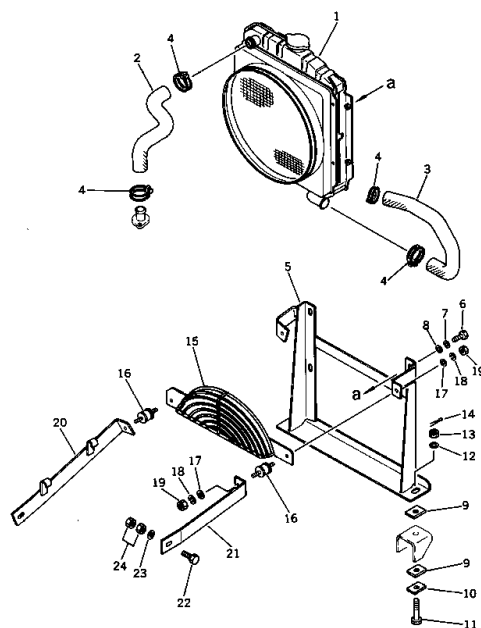
ラジエータ Fig. 1131 RADIATOR (適用 号 機 Serial No. 2001~2259)
