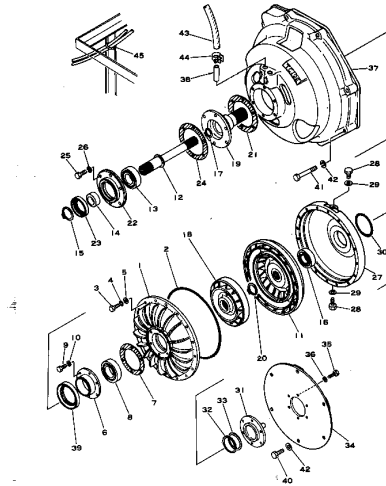
トルクコンバータ Fig. 222 TORQUE CONVERTER (CD25)
