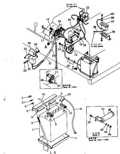
エレクトロニカル システム Fig. 162 ELECTRICAL SYSTEM (CD25)
