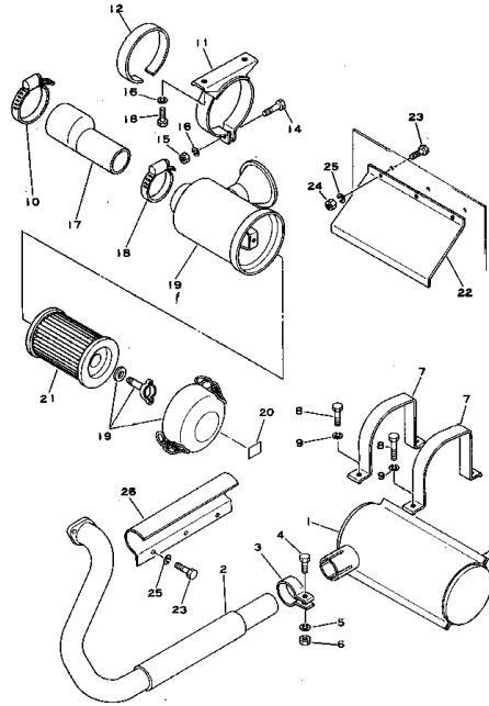
エア インテーク および エキゾースト Fig. 115 AIR INTAKE AND EXHAUST (CD20C)
