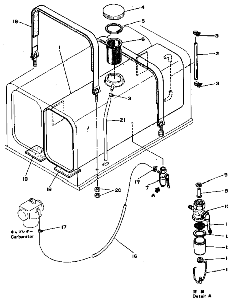
フュエル タンク および パイピング Fig. 141 FUEL TANK AND PIPING (CD20C)
