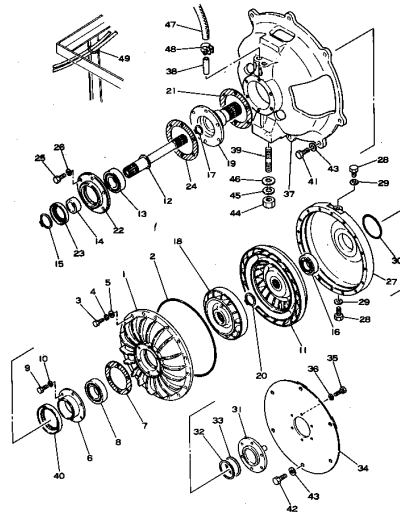
トルクコンバータ Fig. 221 TORQUE CONVERTER (CD20C)
