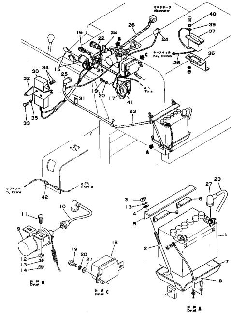
エレクトリカル システム Fig.161 ELECTRICAL SYSTEM (CD20C)
