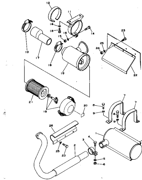
エア- インテーク および エキゾースト Fig. 115 AIR INTAKE AND EXHAUST (CD20)
