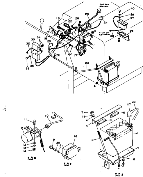
エレクトリカル システム Fig. 161 ELECTRICAL SYSTEM (CD20)
