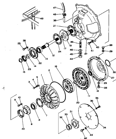
トルクコンバータ Fig. 221 TORQUE CONVERTER (CD20)
