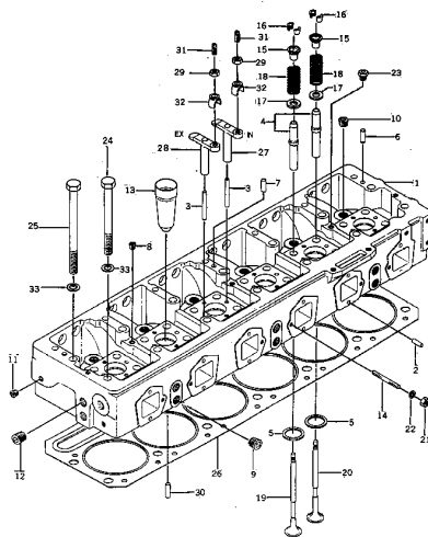
シリンダーヘッド Fig. 101 CYLINDER HEAD
