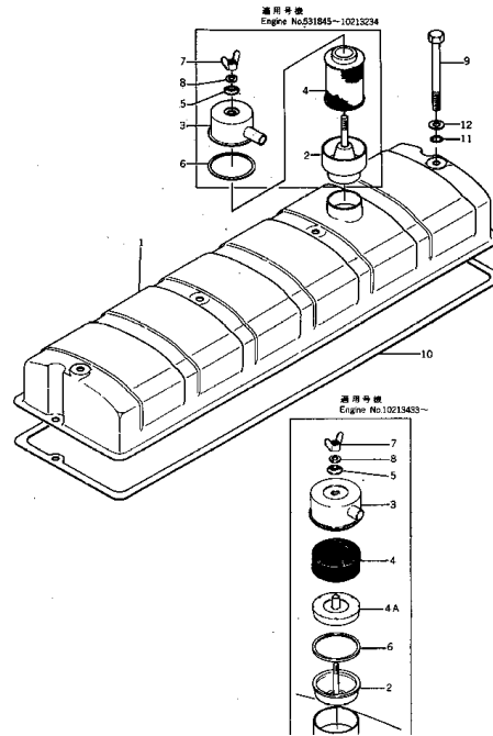
シリンダ ヘッド カバー および ブリーザ Fig. 102 CYLINDER HEAD COVER AND BREATHER
