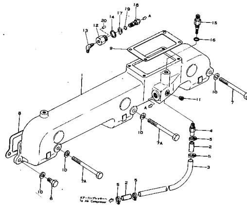
インテーク マニホールド および コネクション Fig 104 INTAKE MANIFOLD AND CONNECTION
