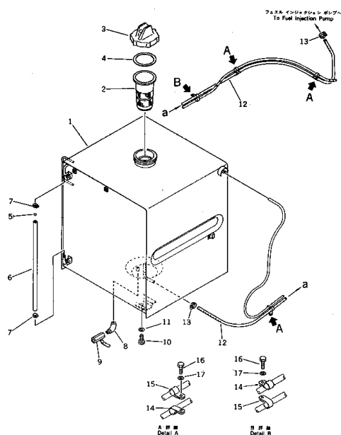
フュエルタンク Fig. 141 FUEL TANK
