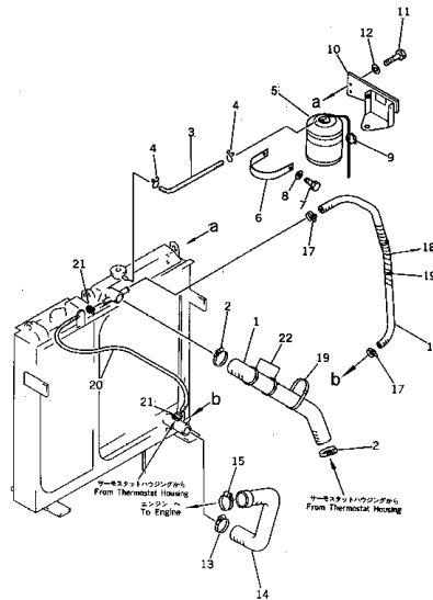
ラジエーターパイピング Fig. 132 RADIATOR PIPING
