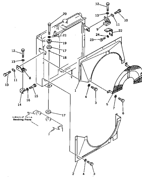
ラジエータ ガード Fig. 133 RADIATOR GUARD
