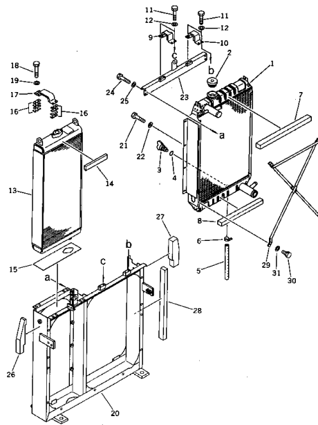
ラジエータ および オイルクーラ Fig. 131 RADIATOR AND OIL COOLER
