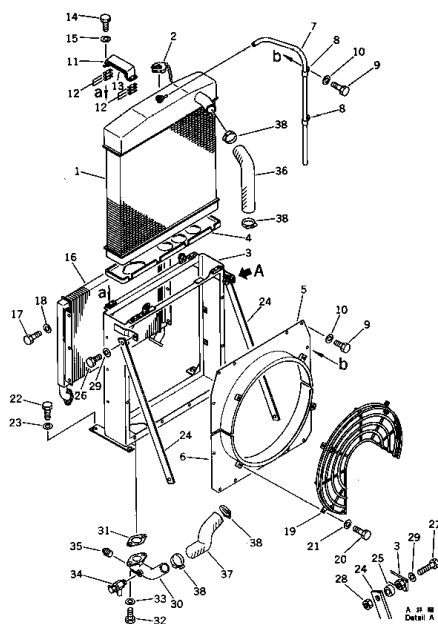
ラジエータ および クーリング Fig. 131 RADIATOR AND COOLING (適用 号 機 (Serial No. 1001~2000))
