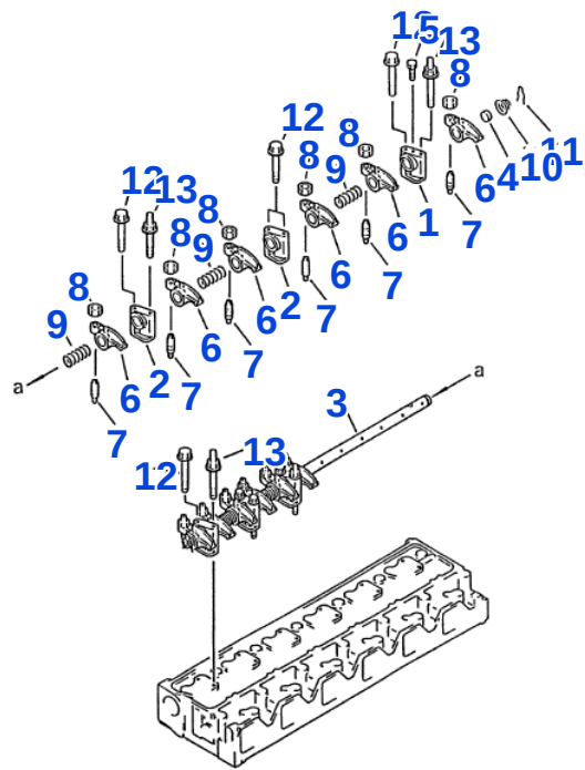
Fig. 103 ROCKER ARM
