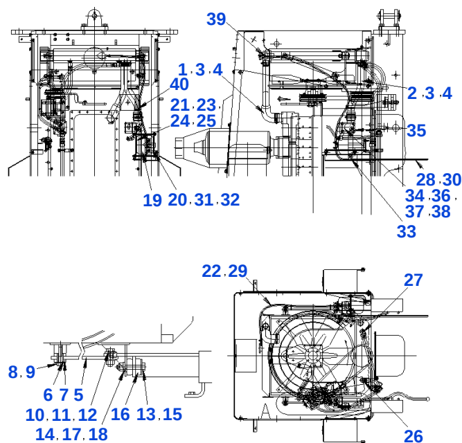
A 詳細 (1:2)
