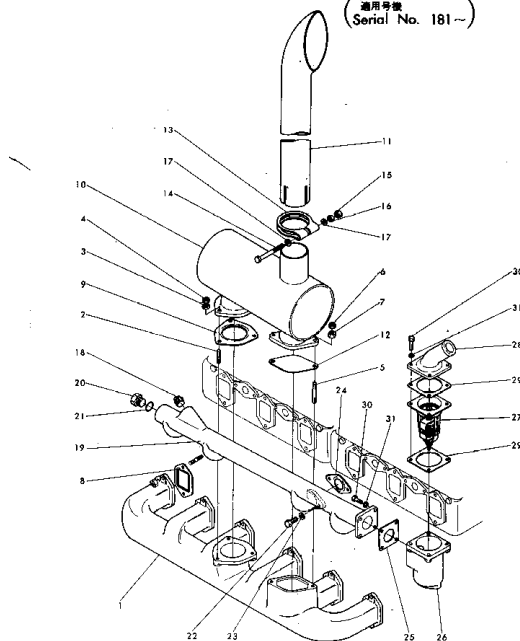
Fig. 105A EXHAUST AND WATER MANIFOLD エキゾースト および ウォータ マニホールド, EXHAUST AND WATER MANIFOLD エキゾースト マフラー および サーマスタット EXHAUST MUFFLER AND THERMOSTAT (適用機種 Serial No. 181~)
