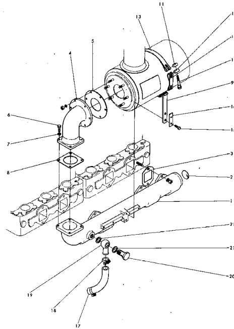
Fig.104A エア インテーク マニホールド (適用機種 Serial No. 233 ~)
