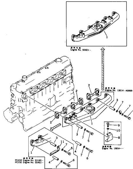
エキゾースト マニホールド FIG. 121 EXHAUST MANIFOLD
