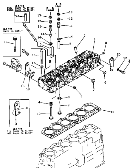
シリンダヘッド FIG. 101 CYLINDER HEAD
