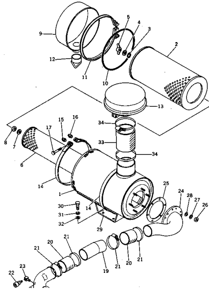
エアー クリーナ 適用 図 FIG. 162 AIR CLEANER (EG80 ENGINE NO. 55458-)
