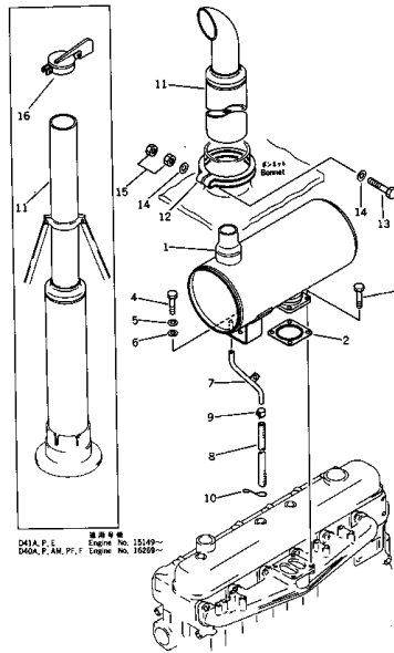
マフラー 適用機種 FIG. 184 MUFFLER (EG80 ENGINE NO. 55458-57709)
