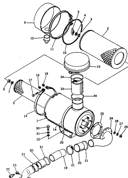
エアー クリーナ FIG. 162 AIR CLEANER
