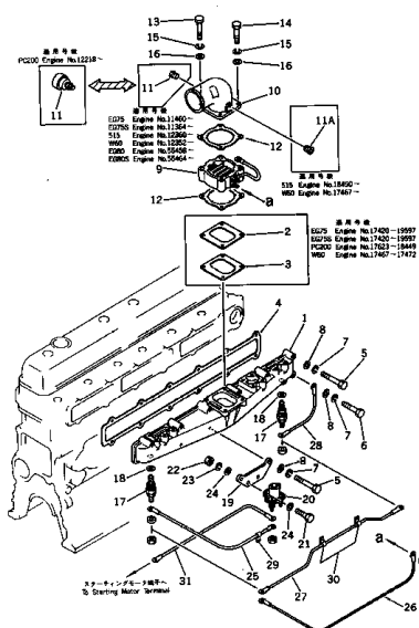
エア インテーク マニホールド および コネクション FIG. 113A AIR INTAKE MANIFOLD AND CONNECTION (EG75 ENGINE NO. 17420-) (EG76S ENGINE NO. 17420-) (EG76S ENGINE NO. 17420-)
