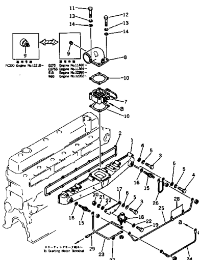
エア インテーク マニホールド および コネクション FIG. 113 AIR INTAKE MANIFOLD AND CONNECTION 適用機種 (EG75 ENGINE NO. 11460-17419) (EG75S ENGINE NO. 11364-17419)
